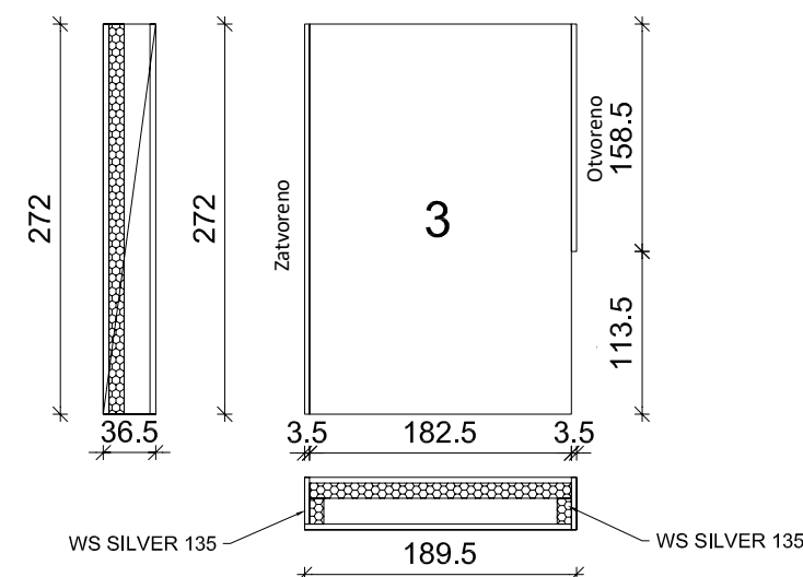
Primjer nacрте montažnih modula.
