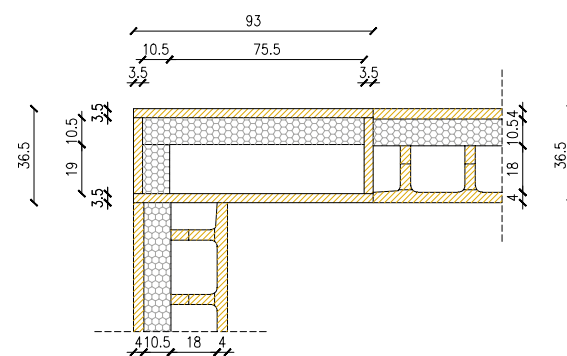
ŠIROKI STUP (primjena na kutnim dijelovima) 19cmx76cm, debljina bloka 36,5 cm, s vanjskom izolacijom od 10,5 cm i bočnom izolacijom od 10,5 cm, od EPS-a s GRAFITOM + 3,5 drvobetona
