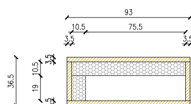
ŠIROKI STUP (kutni dijelovi) 19cmx76cm, debljina bloka 36,5 cm, s vanjskom izolacijom od 10,5 cm i bočnom izolacijom od 10,5 cm, od EPS-a s GRAFITOM + 3,5 drvobetona
