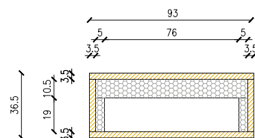
ŠIROKI STUP 19cmx76cm, debljina bloka 36,5 cm, s vanjskom izolacijom od 10,5 cm i bočnom izolacijom od 5 cm, od EPS-a s GRAFITOM + 3,5 drvobetona
